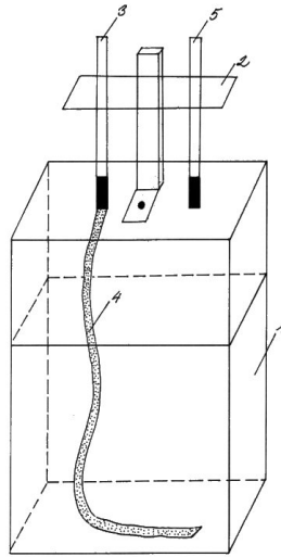
Obr. 2 Augustův psychrometr kazetový (vyrobený a užívaný v OVM v Šumperku)
